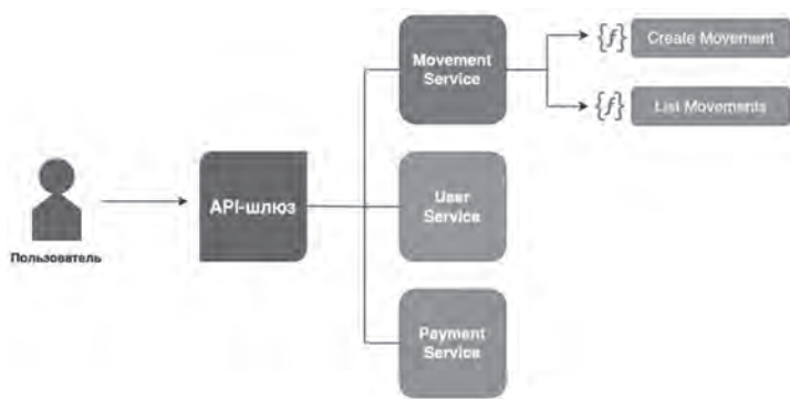
Рисунок 6. Микросервисная Serverless-архитектура
