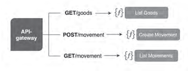
Рисунок 3. Работа API-шлюза
