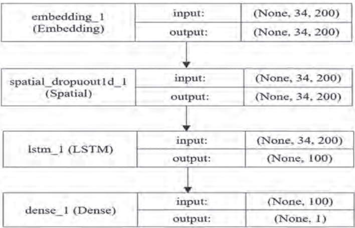
Рисунок 6. Архитектура рекуррентной сети
